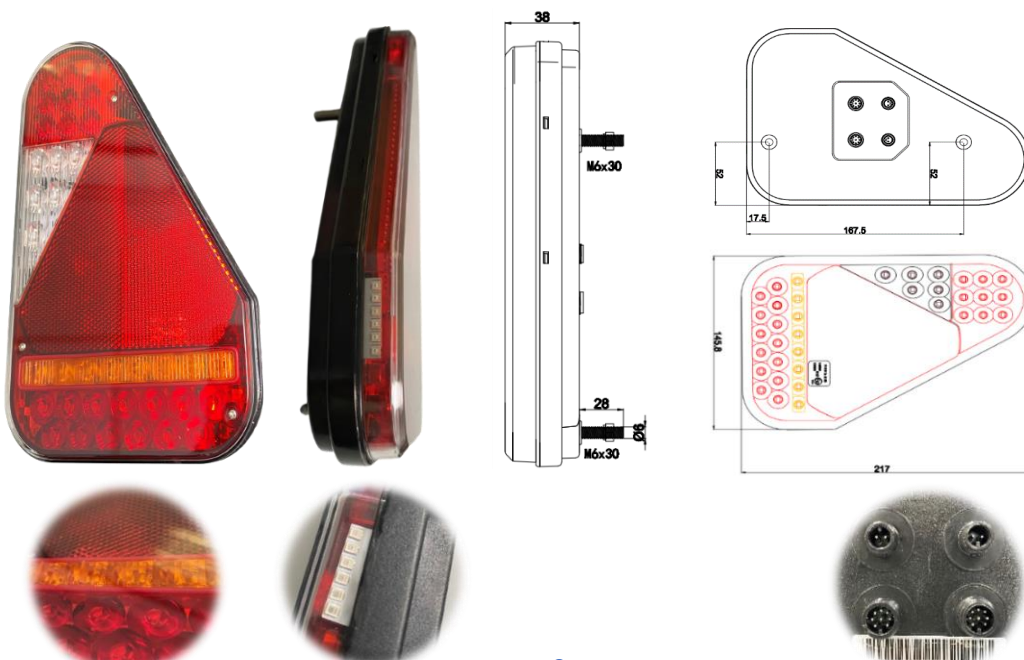
Feux LI® 6 : 2x8C F + 2x2C F
